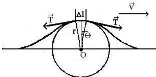
Figura 1. Representação de um pulso que se propaga ao longo de uma corda.
